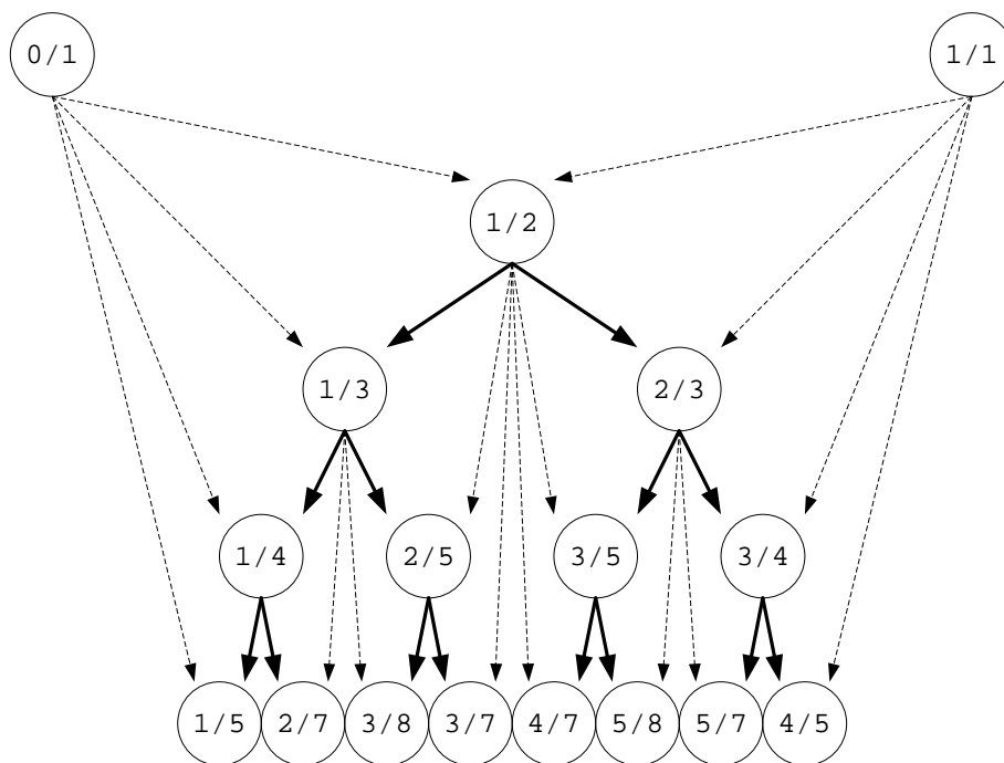
スターン・ブロコット木(Stern-Brocot Tree)の一部 (『コンピュータの数学』p.116の図を元に結城が作成)
